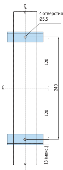
Монтажный чертёж
