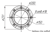
Фланцы переходника для: 31В 10-120, 31В 10-160, 31В 12-160, 31В 12-210, 31В 12-250
